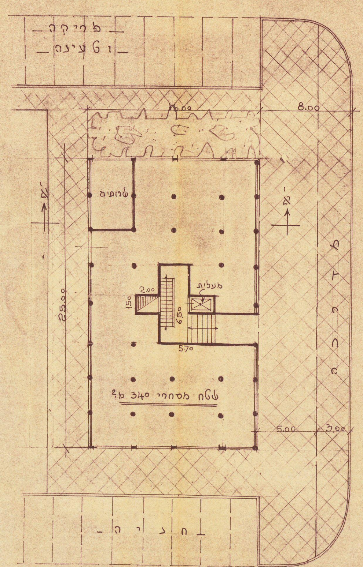
תכנית הקומה הסטנדרטית ק.מ. 1:200
