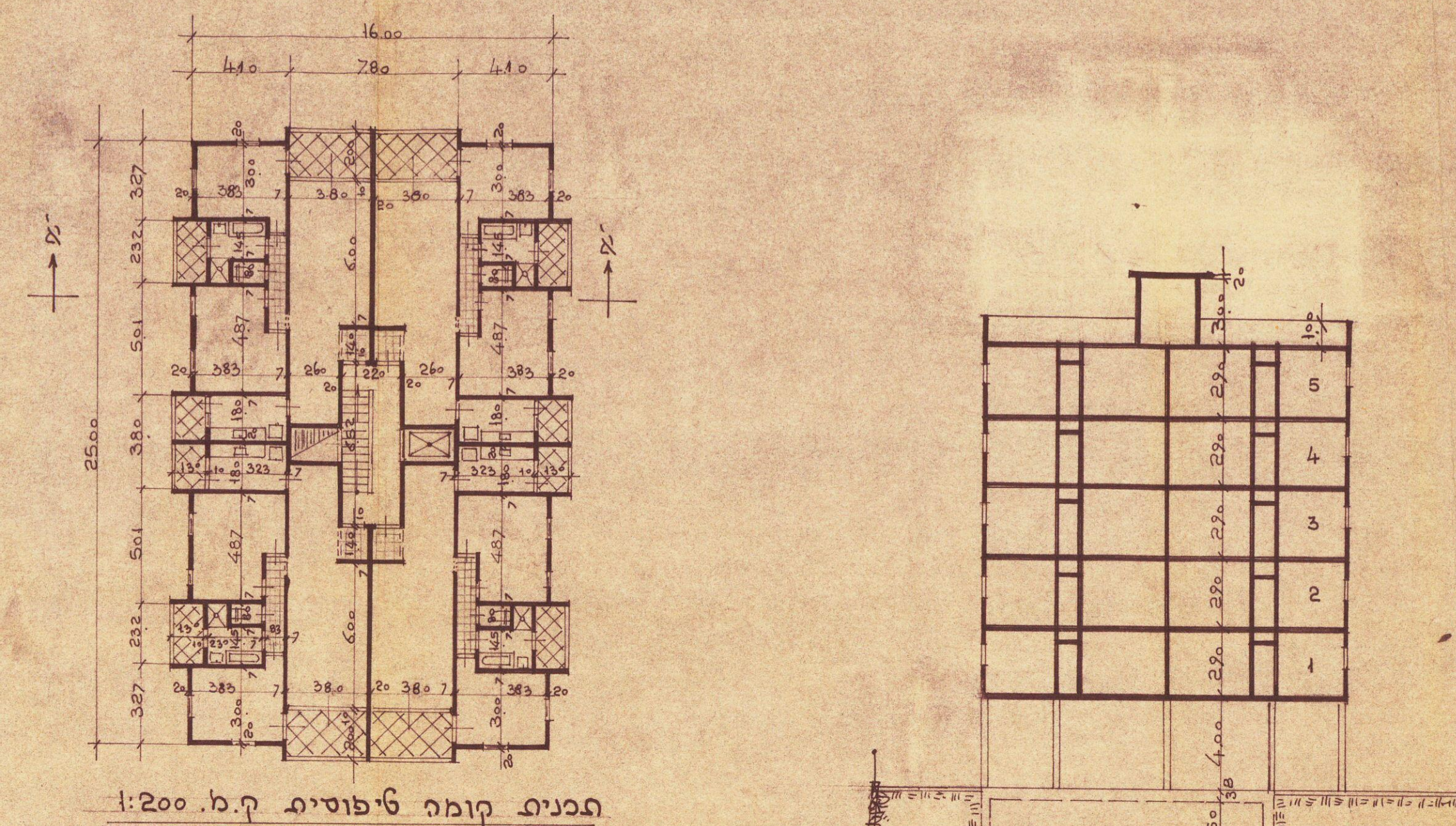
תכנית קומה טיפוסיית ק.מ. 1:200
