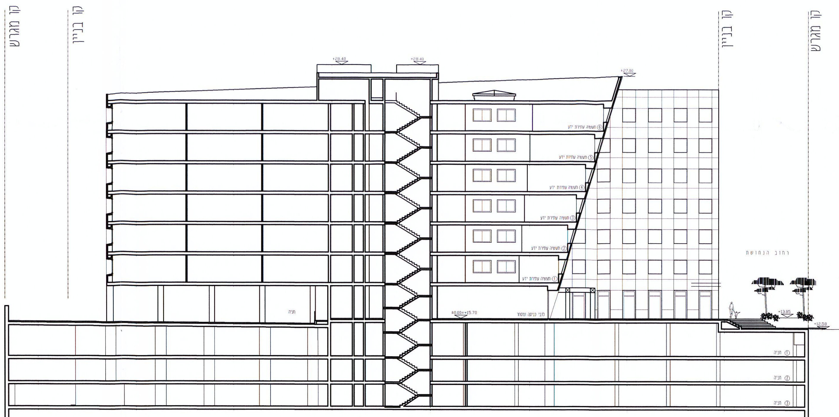
חתך אורך קנ"מ 1:250
