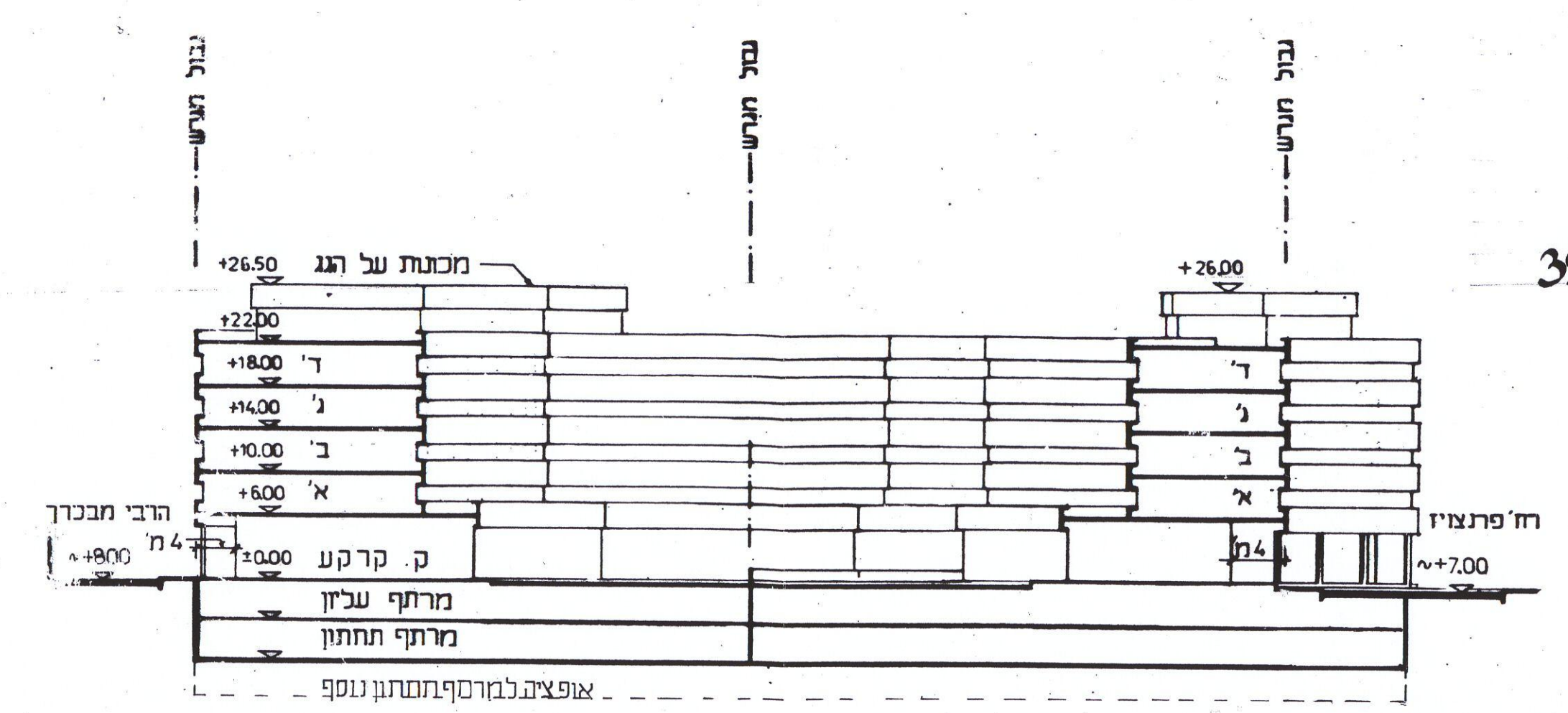
חתך א-א 1:500
