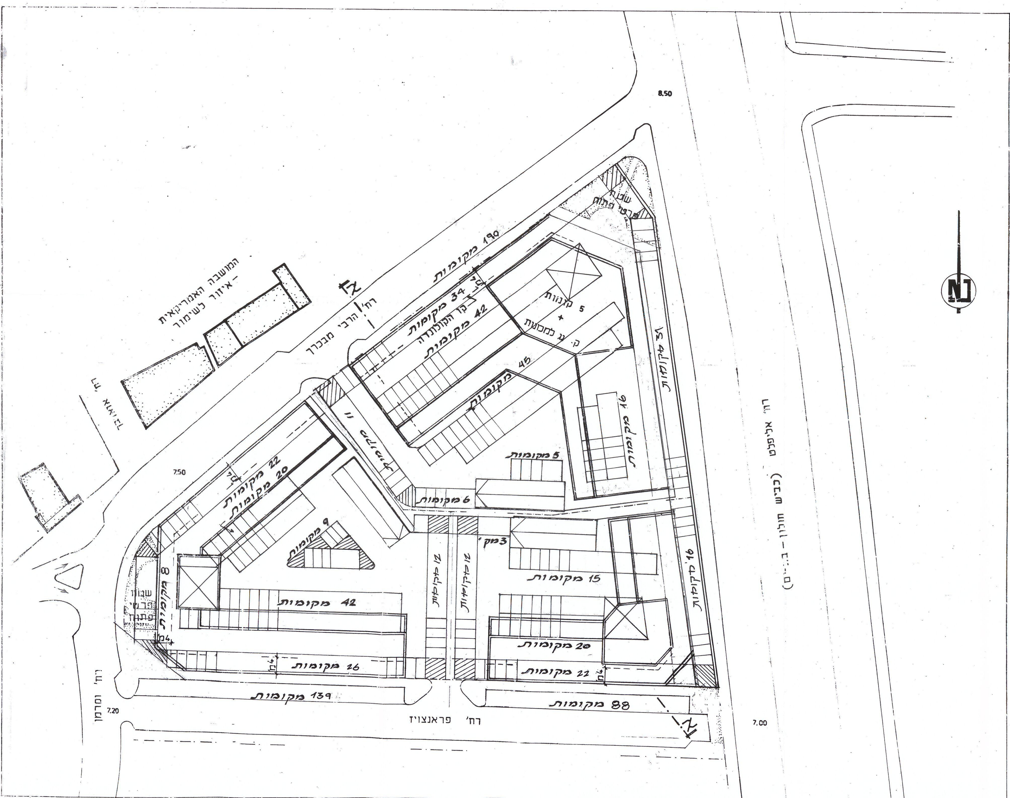
תכנית חניה קומת מרתף 1:500
