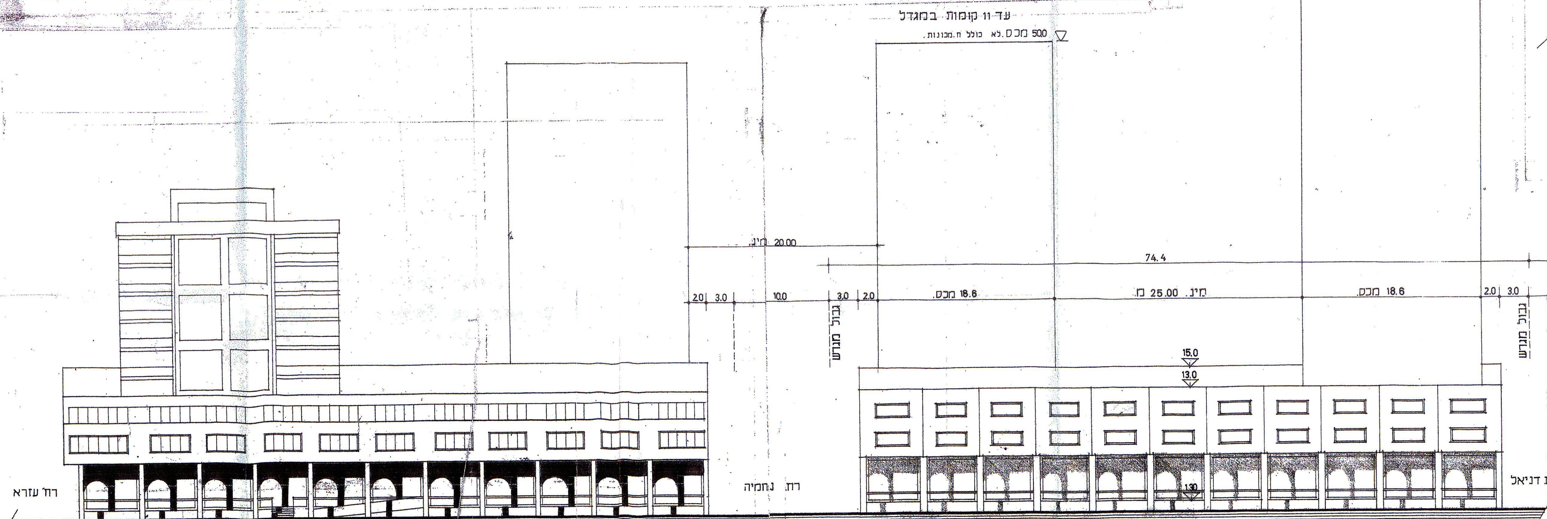
חזית רטיונית להרברט סמואל קו"מ 1:250
