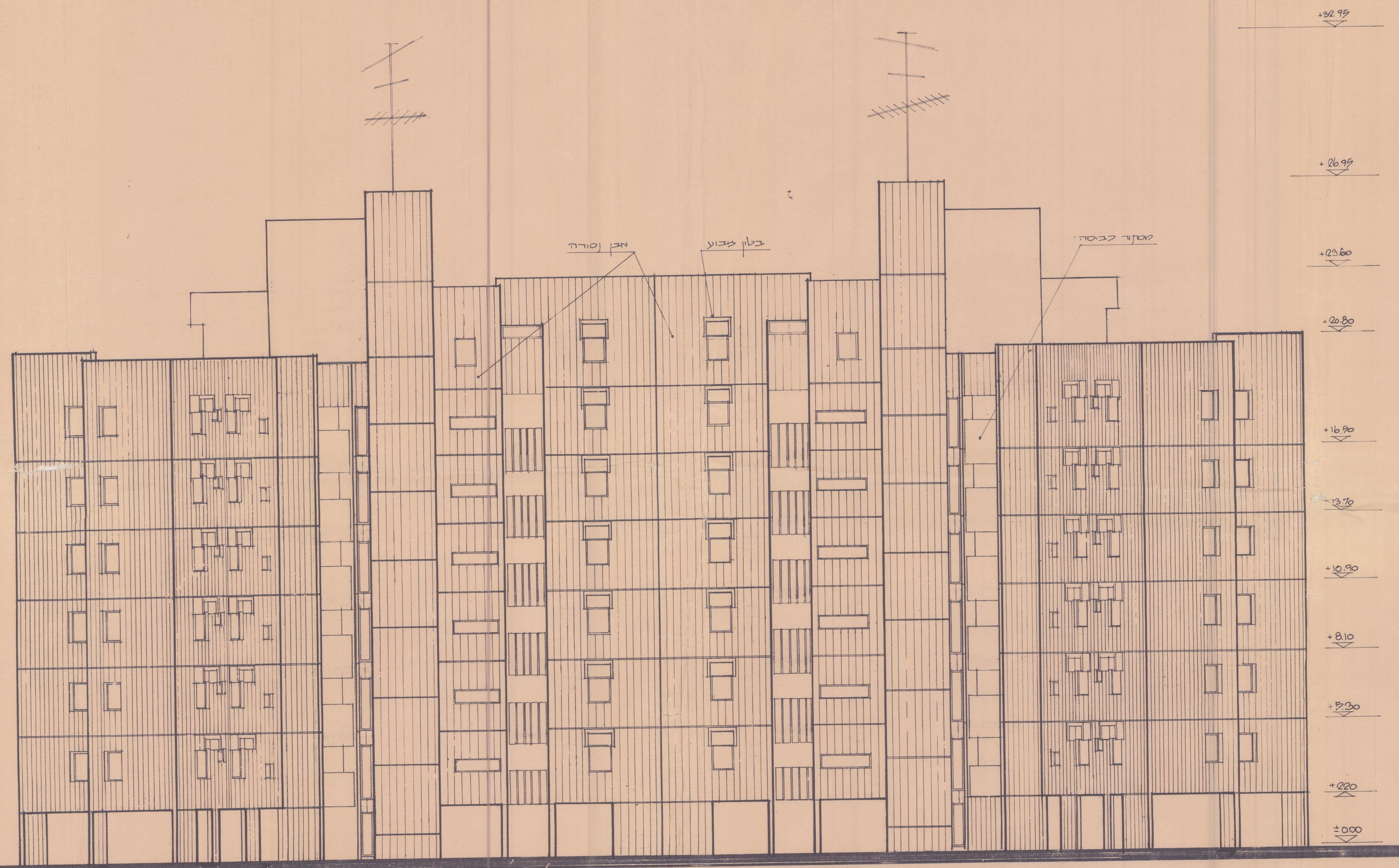
חזית צפונית ק.ב.מ. 1:100
