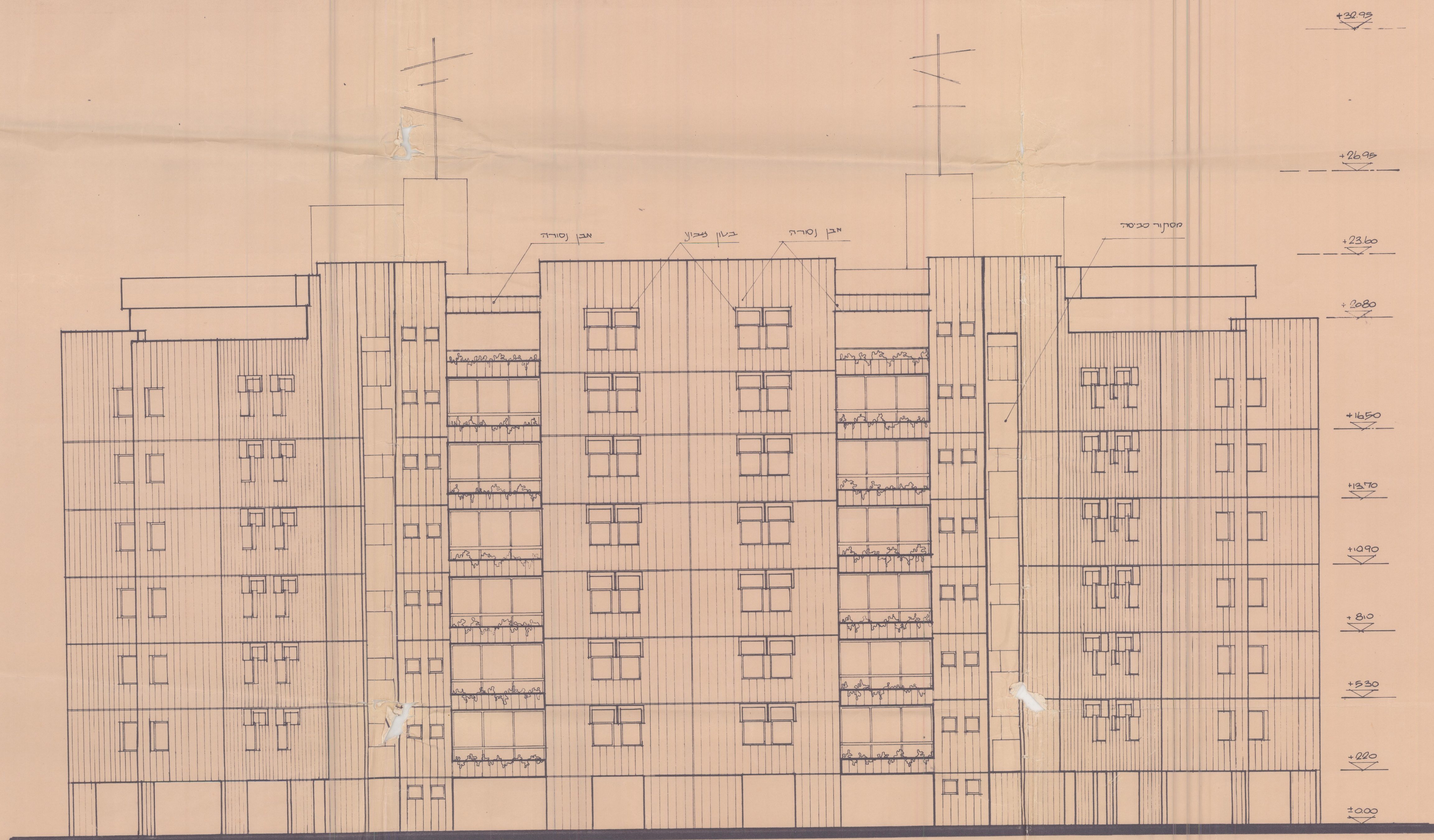
חזית דרומית ק.ב.מ. 1:100
