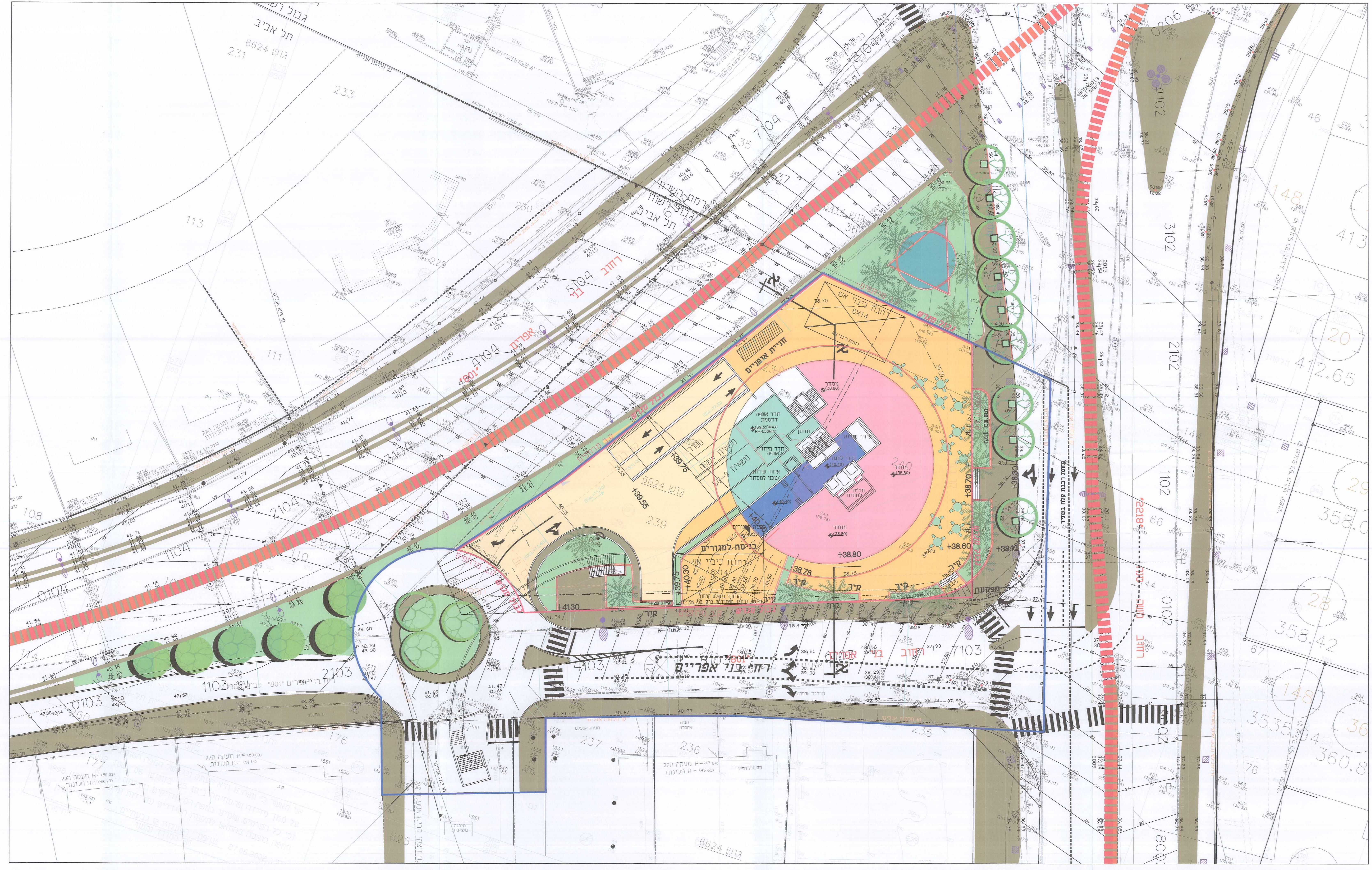
תכנית פיתוח עם שיקוע מתוכנן בצומת הפיל 1:250
