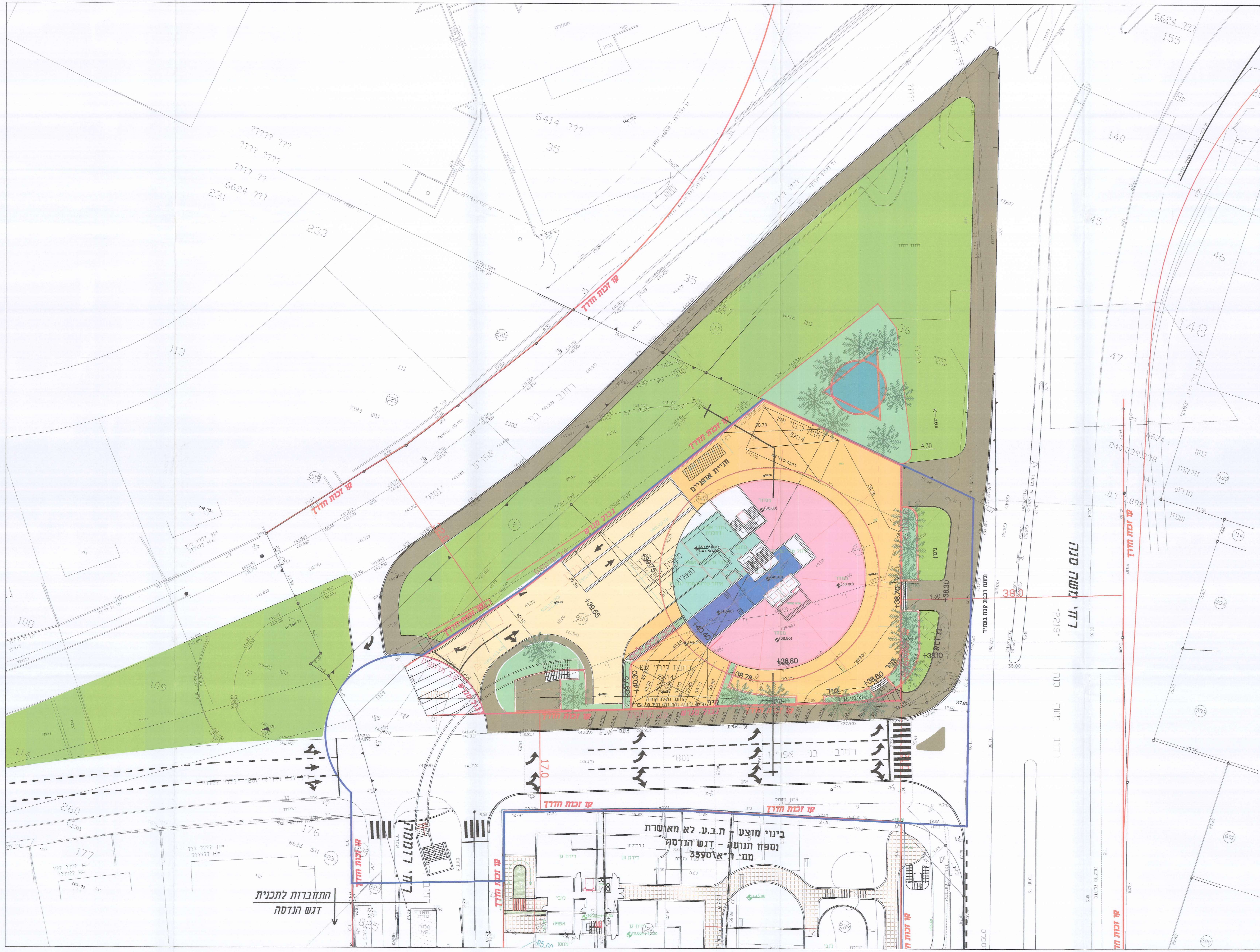
תכנית פיתוח התחברות לקיים 1:250
