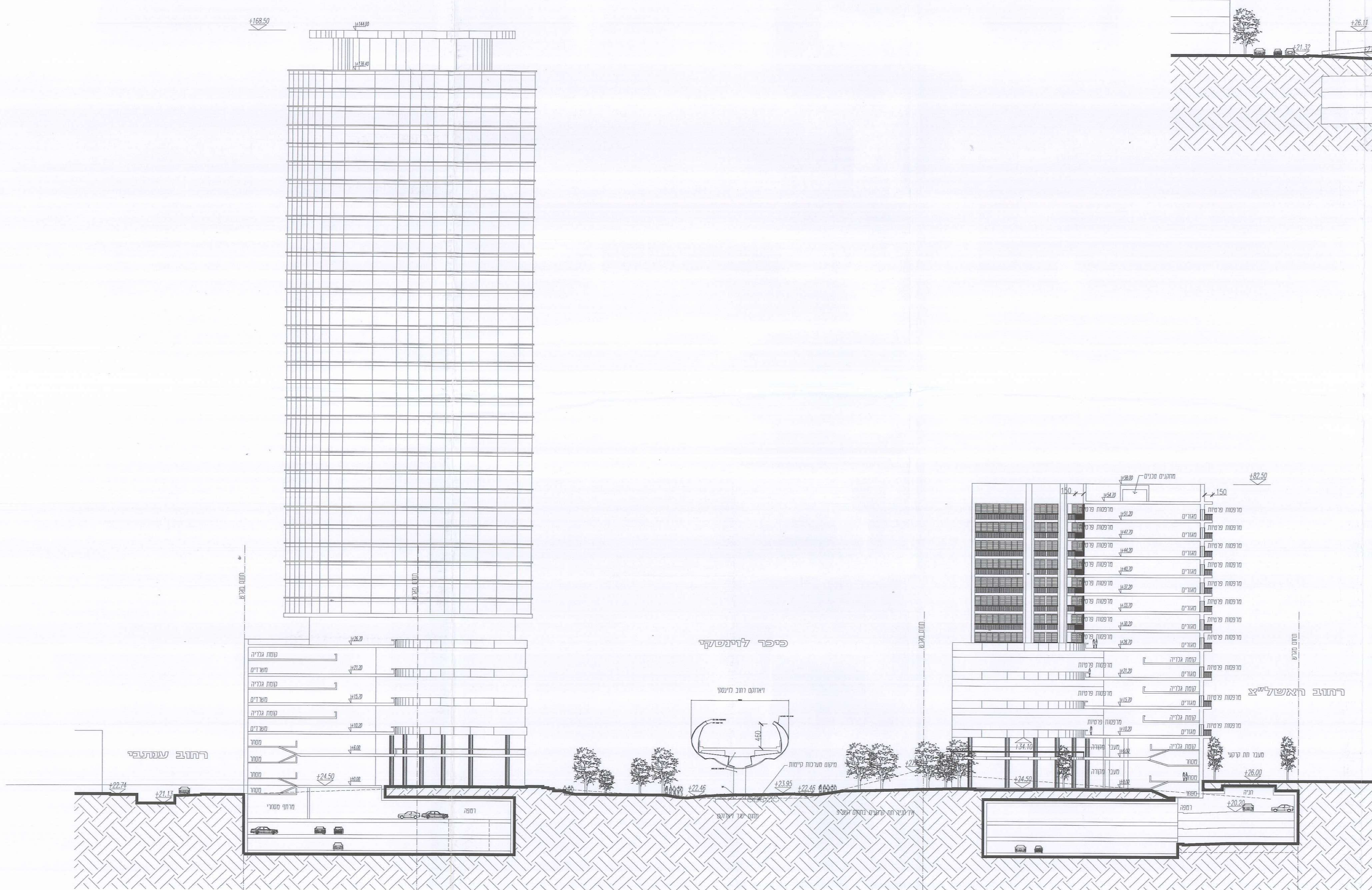
תתק א-א צפון דרום לרוחב הפיכר ק.מ. 1500
