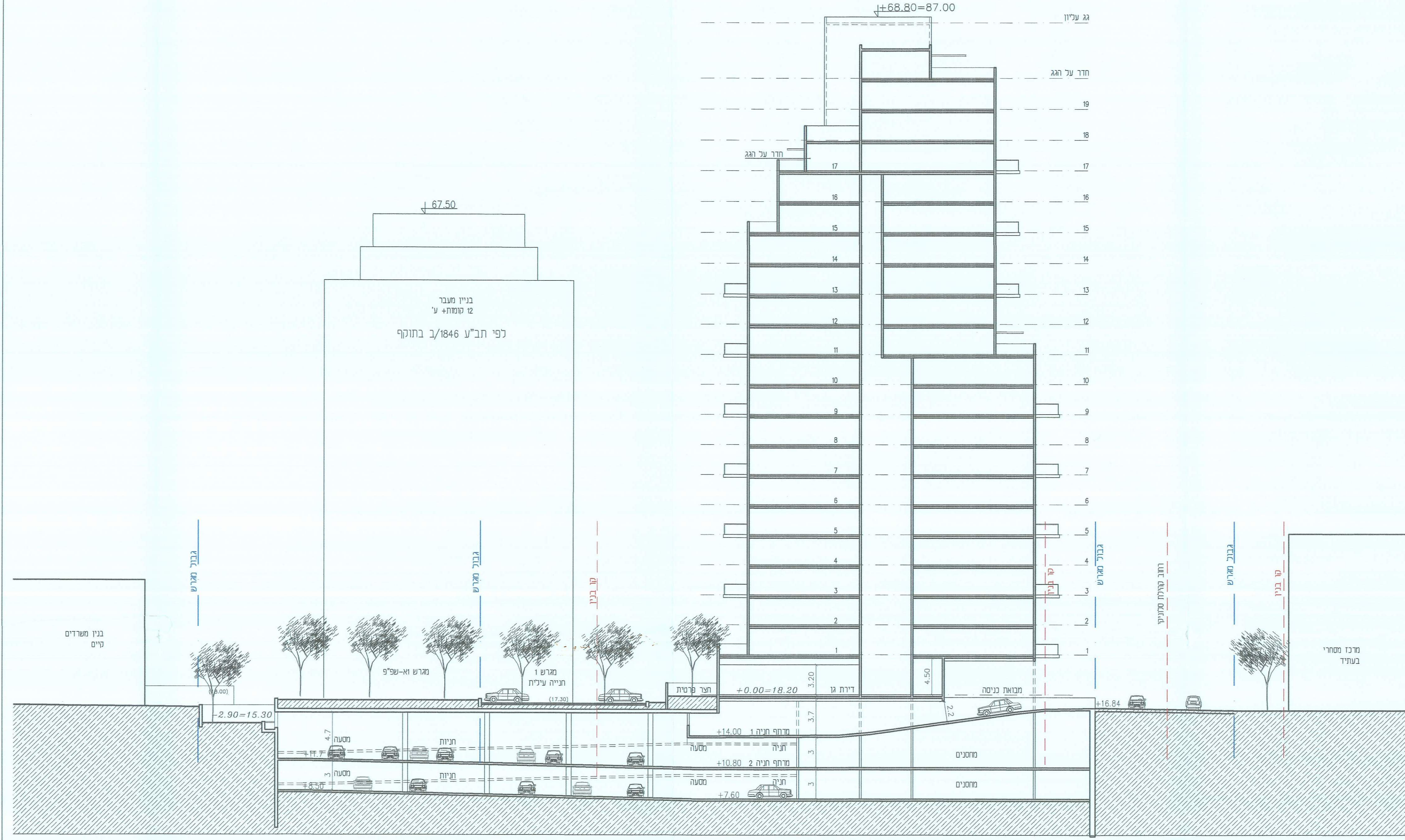
חתך עקרוני בכיוון מזרח-מערב קנ"מ 1:250
