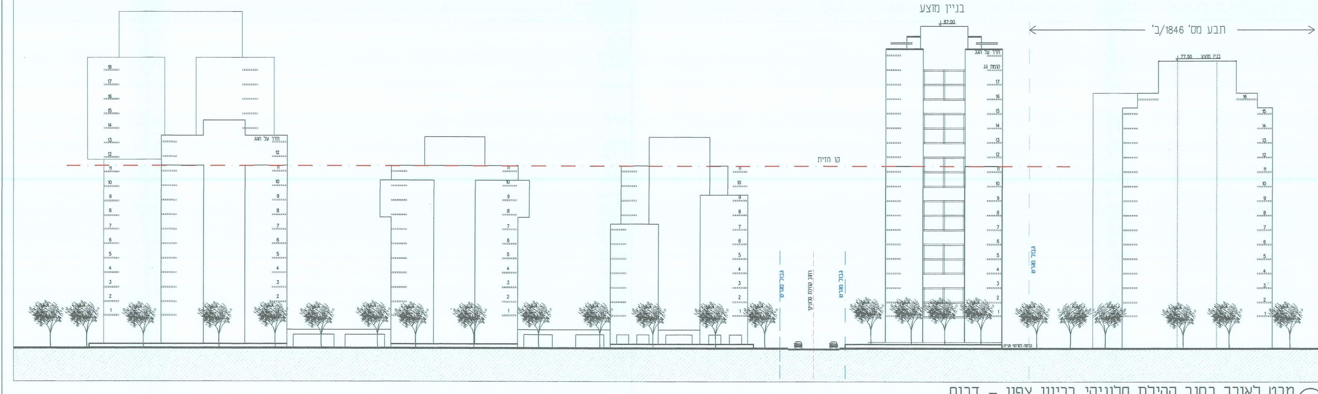
מבט לאורך רחוב קהילת סלונקי בכיוון צפון - דרום קנ"מ 1:500
