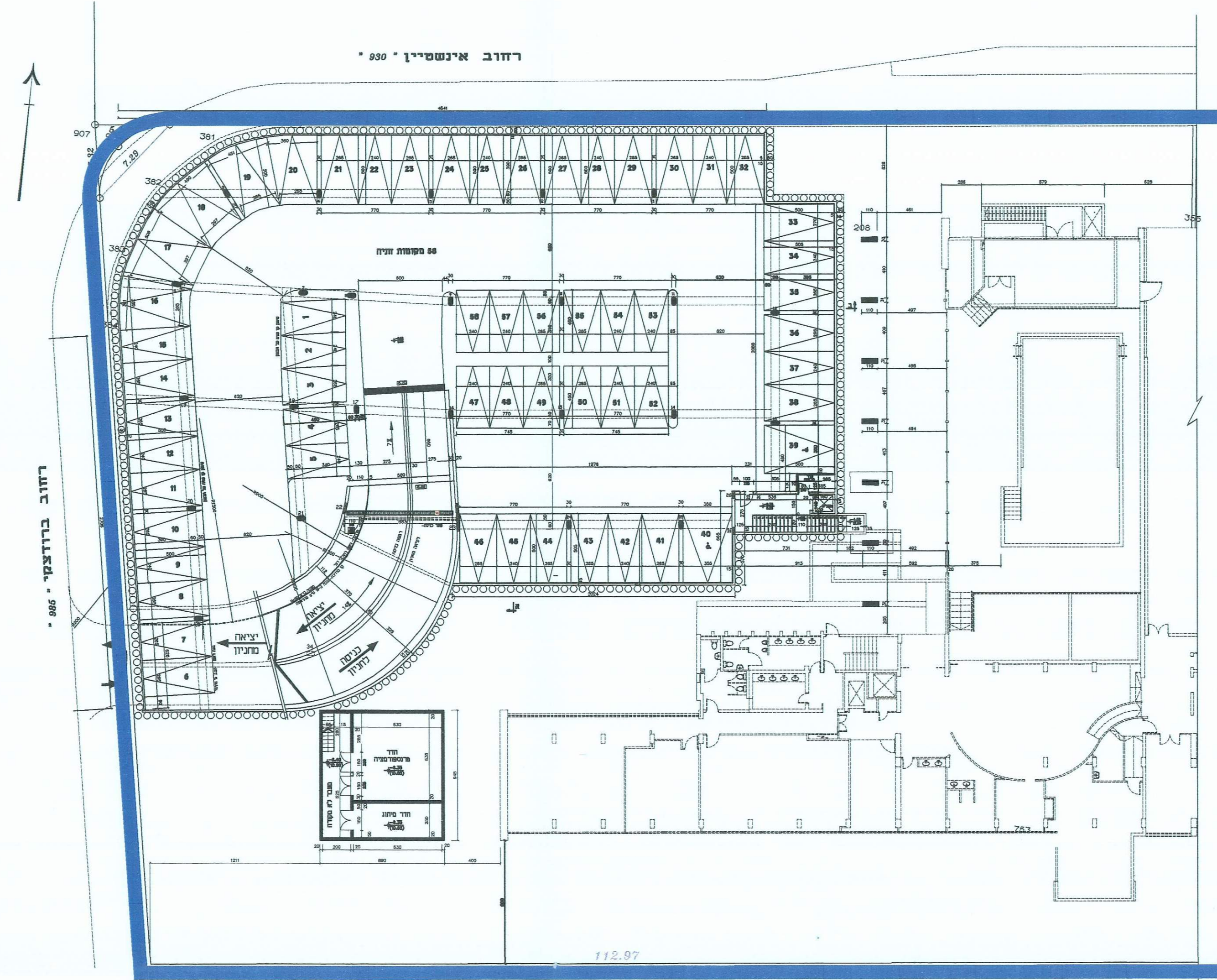
תוכנית קומת מרתף חדש ( מפלס -8.80 ) קנ"מ 1:250
