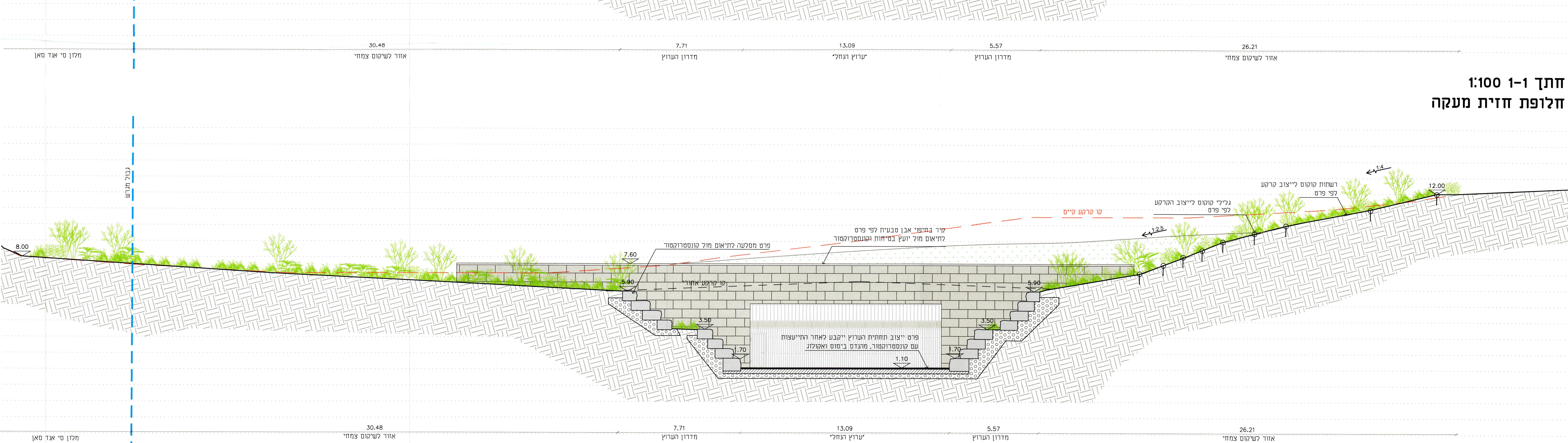
חתך 1-1 1:100 חלופת חזית קיר בגובה 1.1 מ'
