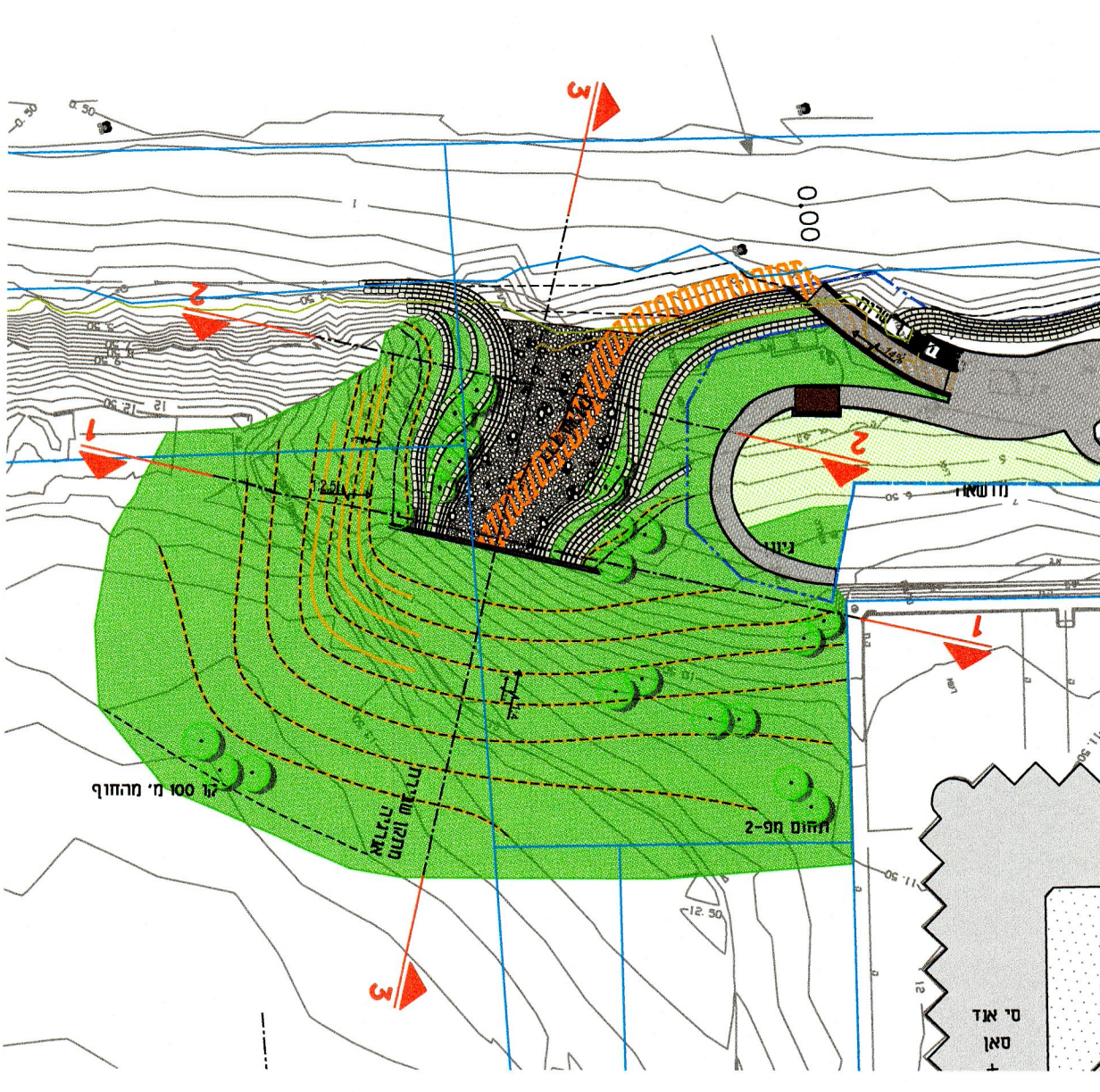
תכנית סביבה 1:1,000
