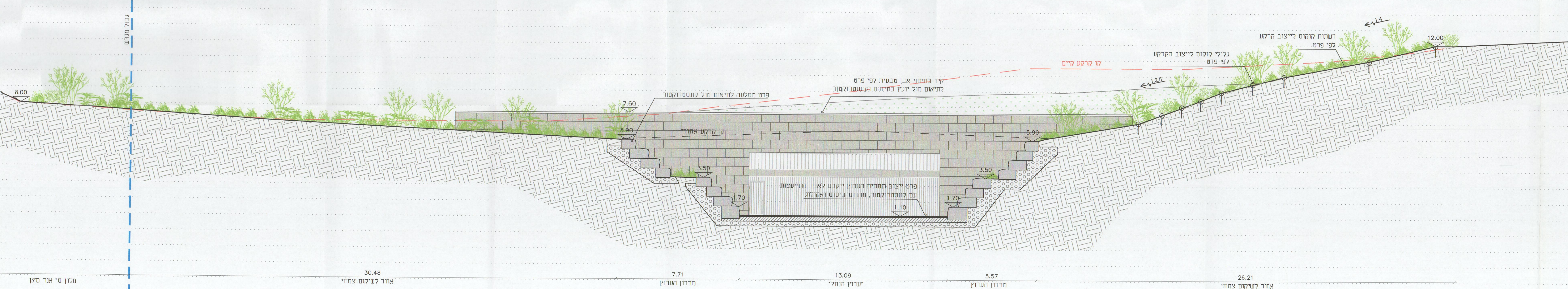
חתך 1-1 1:100 חלופת חזית קיר בגובה 1.1 מ'
