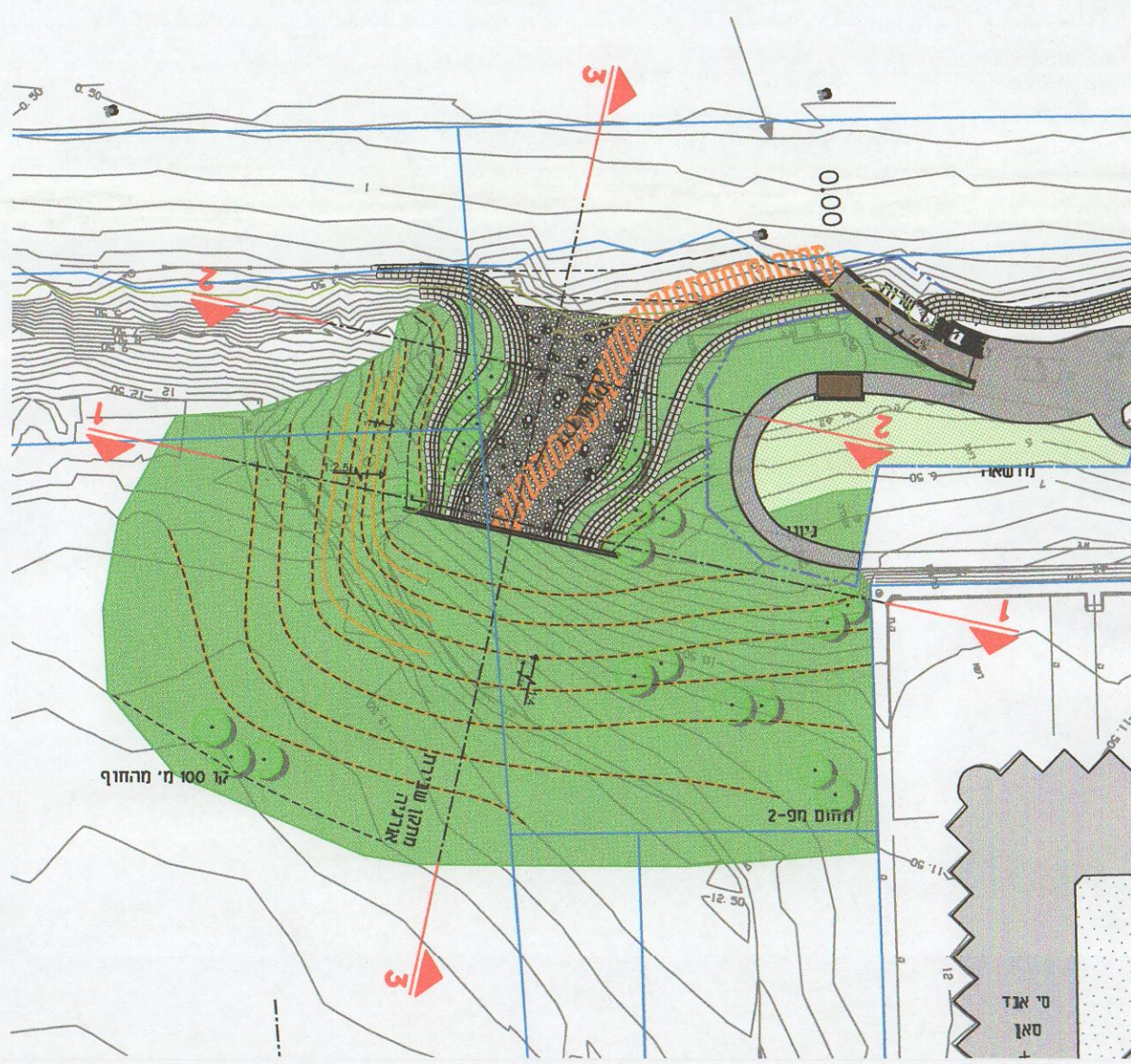
תכנית סביבה 1:1,000
