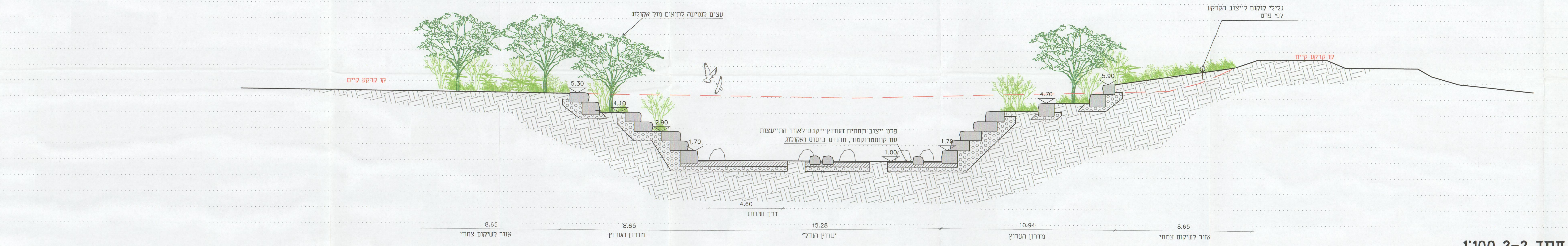
חתך 2-2 1:100
