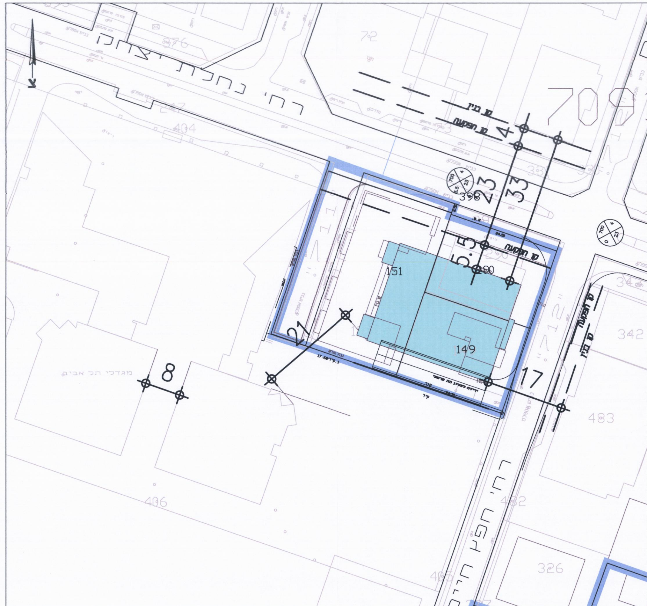
תכנית סביבה: מרחק מבניינים סמוכים, קנ"מ 1:500
