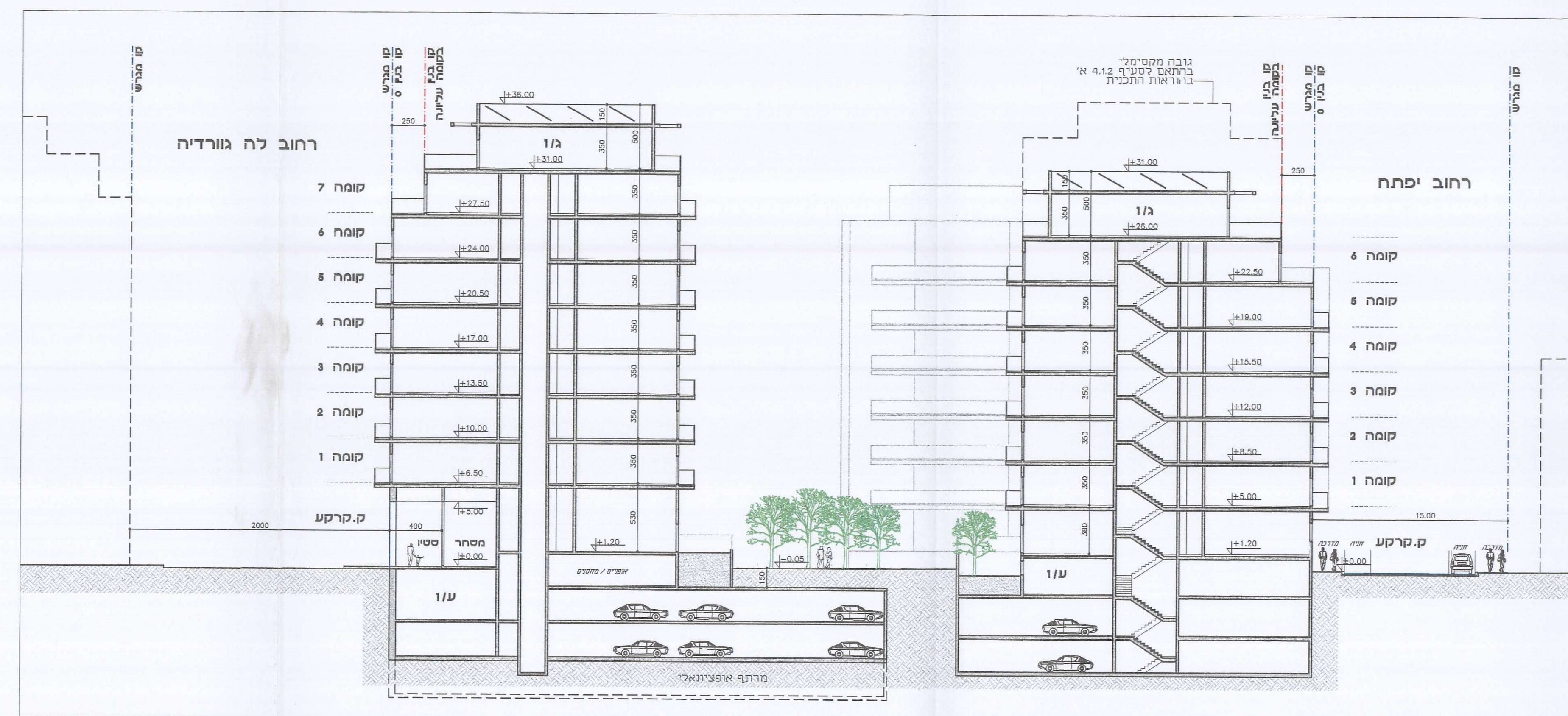
1:250 א-א תת
