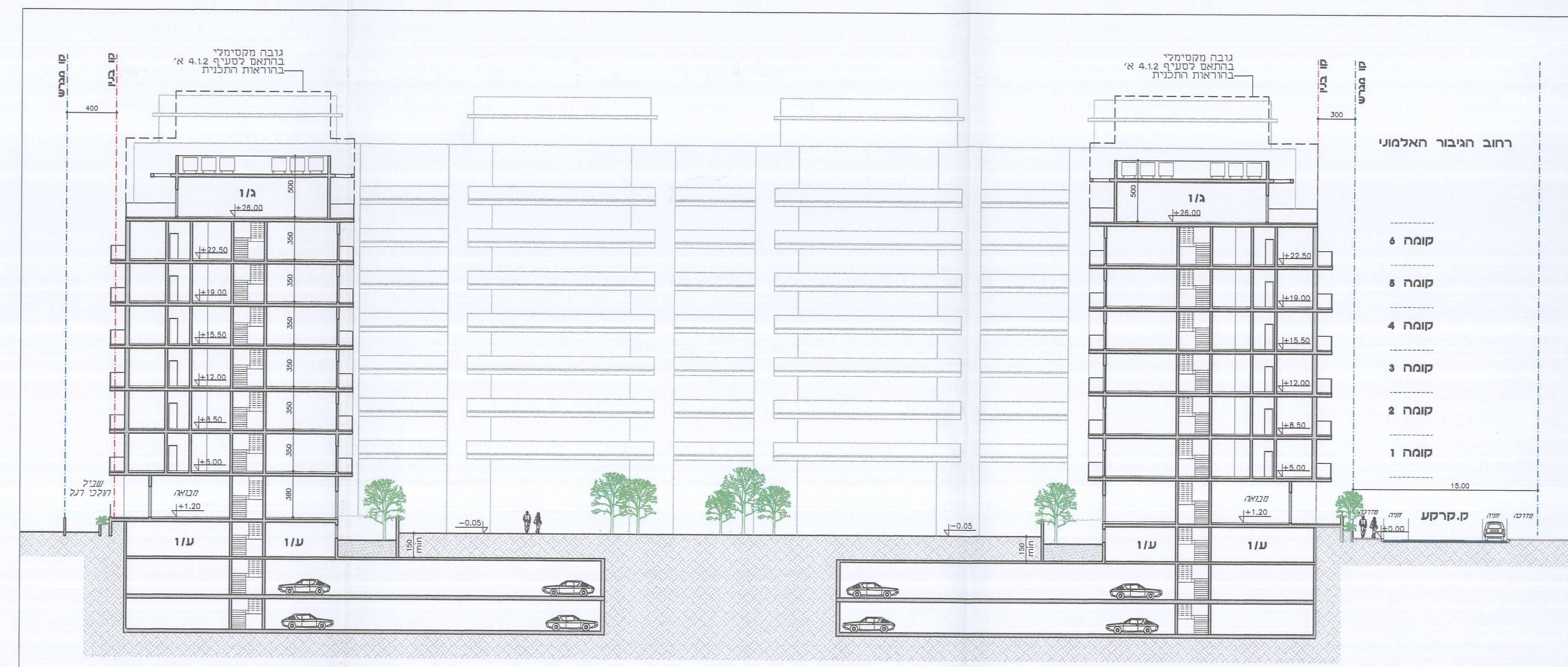
1:250 חתך ב-ב
