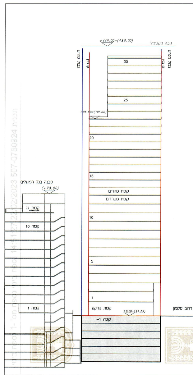
חתך ב-ב 1:1,000
