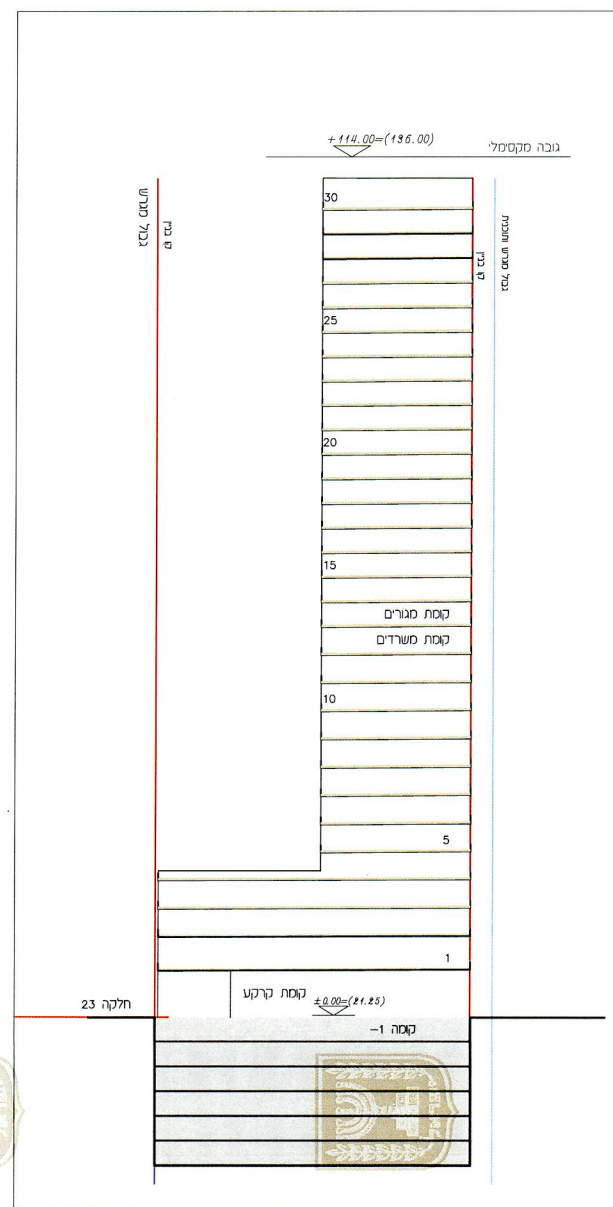
חתך א-א 1:1,000
