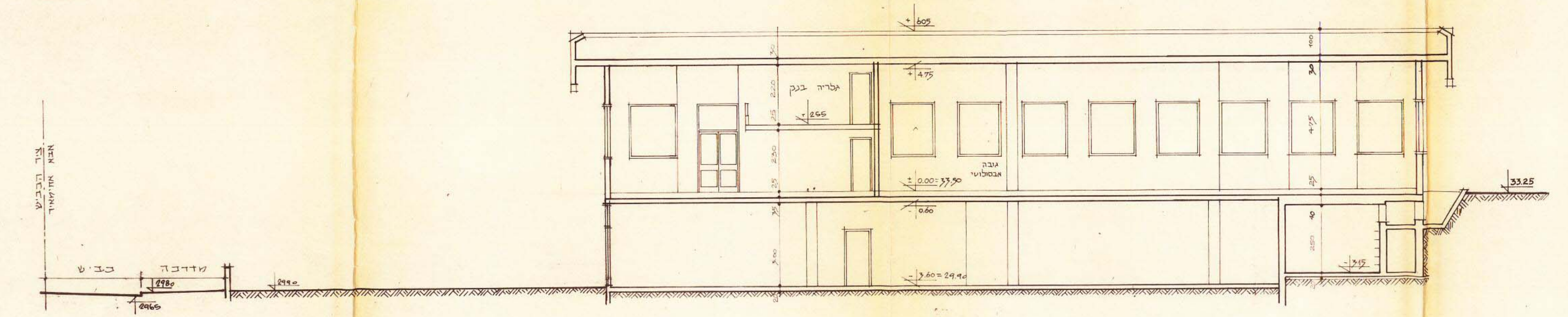
חתך ב-ב
