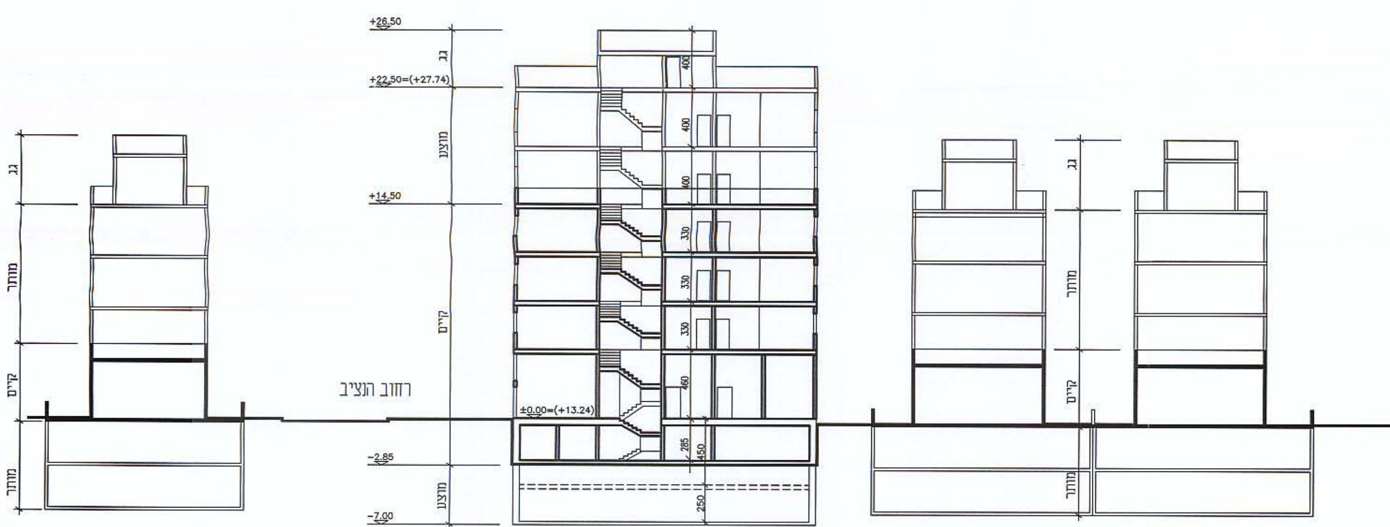
חתך A - A ק.מ. 1:250
