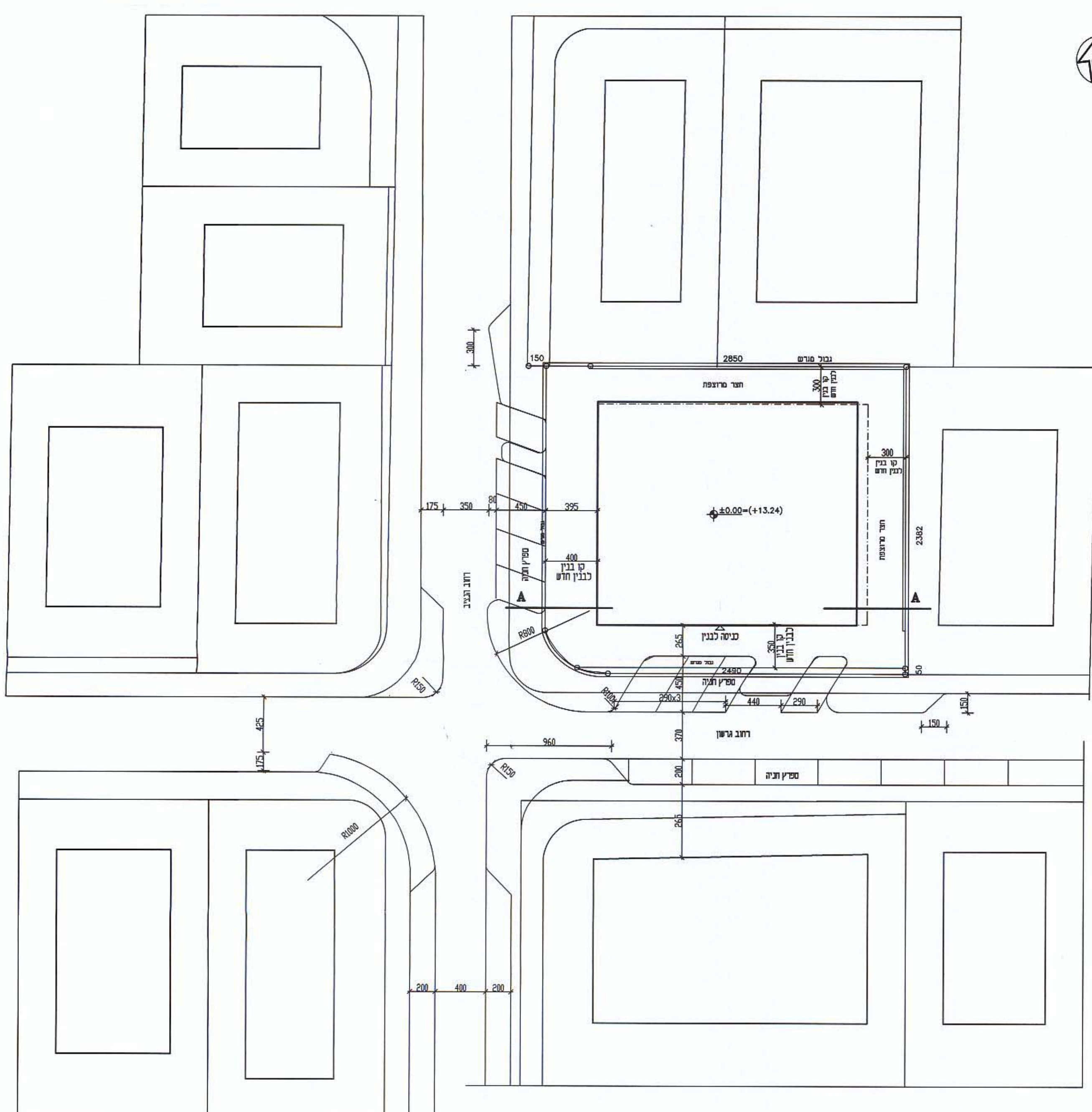
תכנית הבנין ק.מ. 1:250
