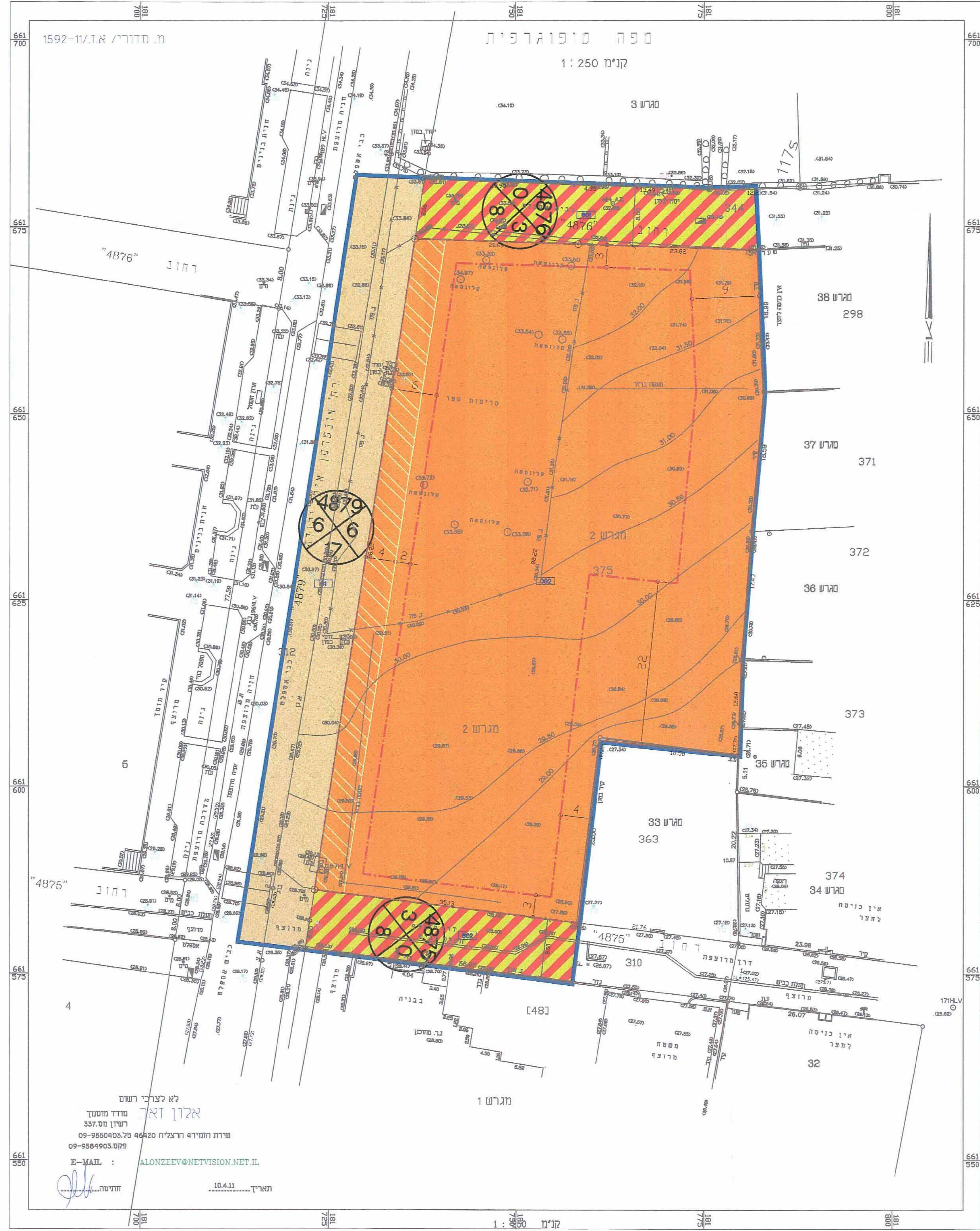
מצב מוצע 1:250
