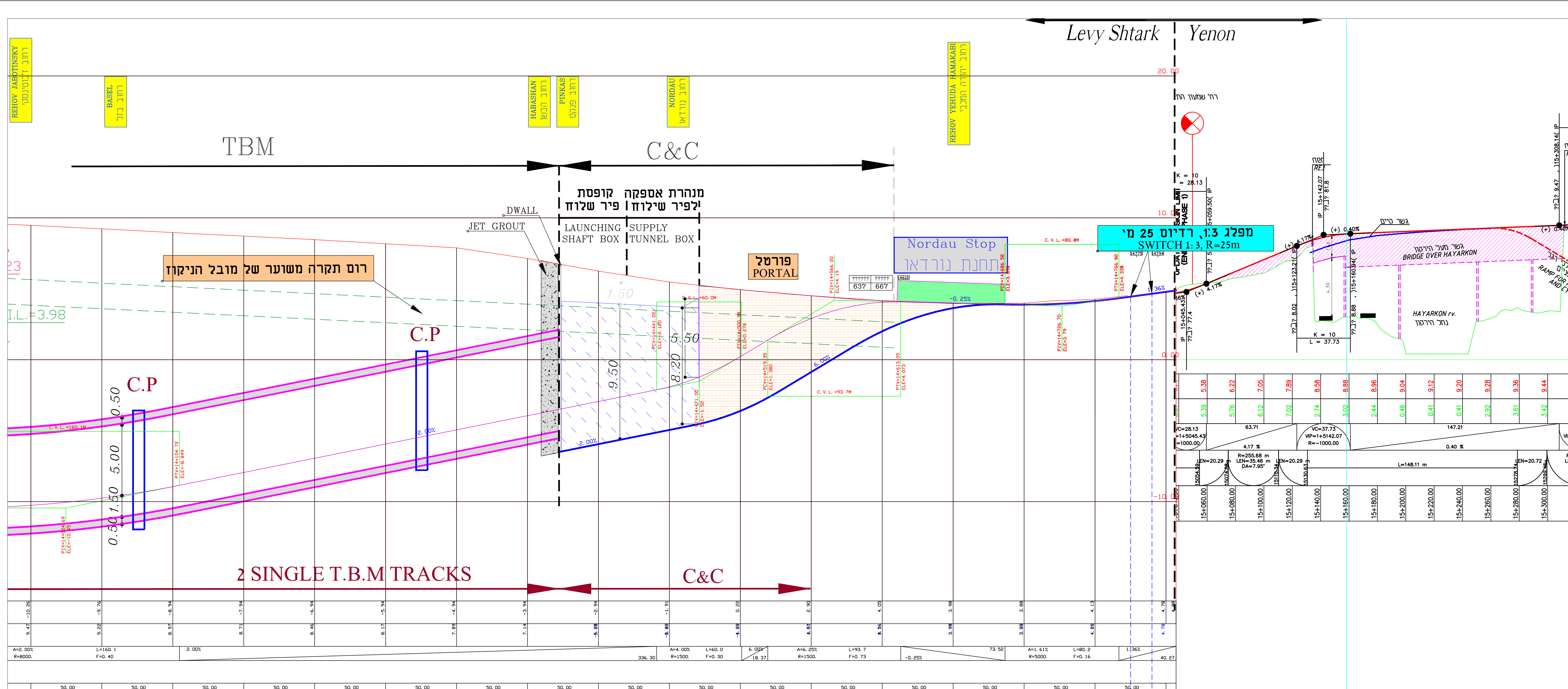
חתך אורך קנ"מ 1:1250
