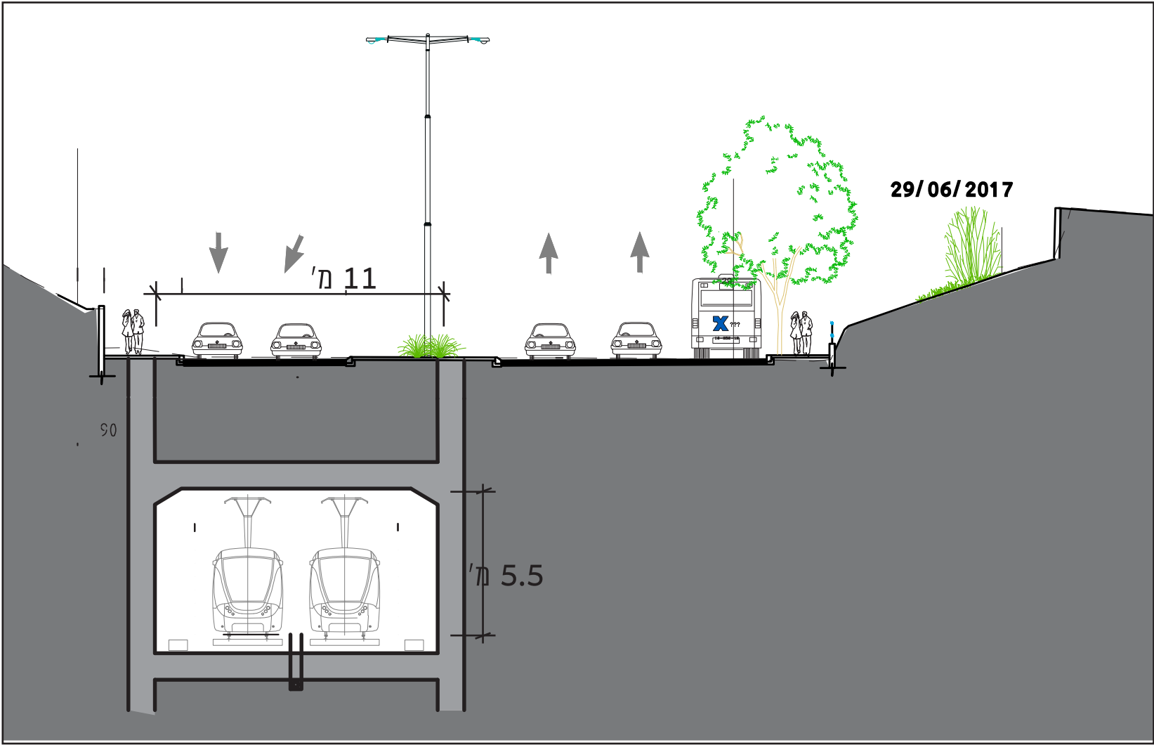
חתך טיפוסי מנהרה
