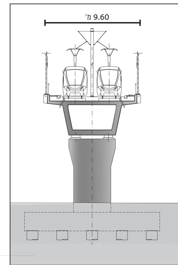
חותך טיפוסי
