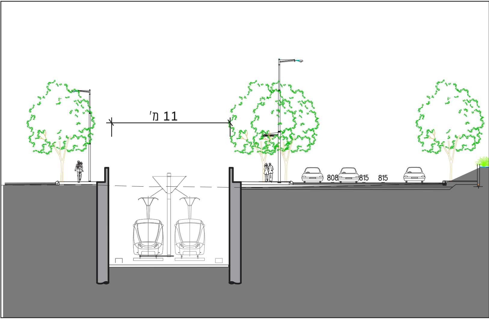
חתך טיפוסי פורטל
